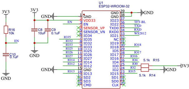
图4 esp32 引脚定义图 Fig. 4 esp32 pinout diagram
