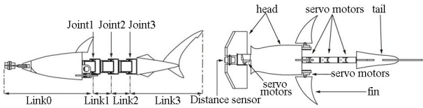
图3 机器鱼结构示意图 Fig. 3 Schematic diagram of the robot fish structure
