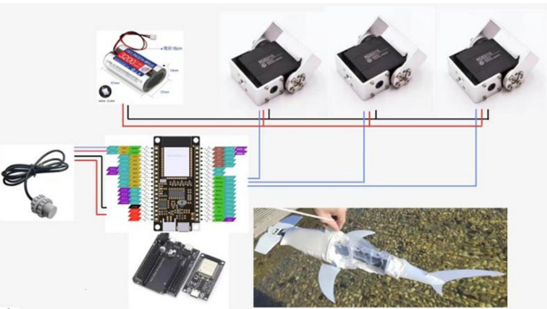
图 5 内部主要电路示意图 Fig. 5 Schematic diagram of the main internal circuits
