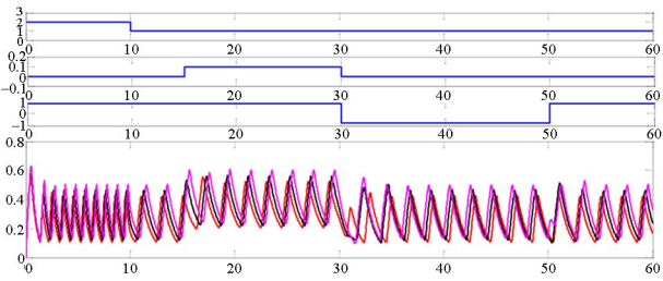
图 9 步态切换示意图 Fig. 9 Gait transition illustration
